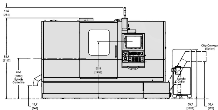
Vorderansicht
