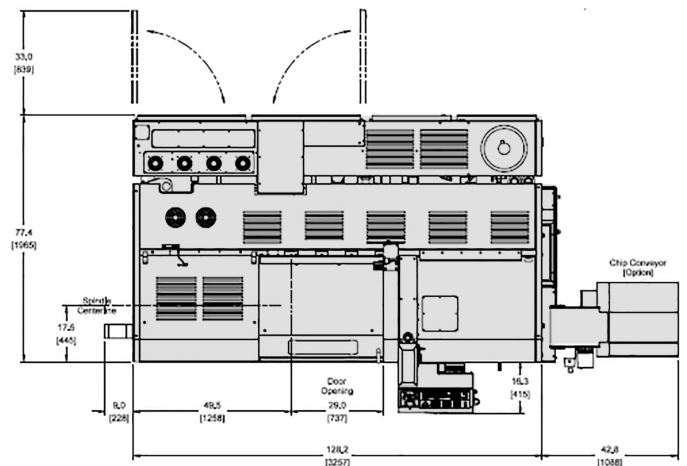
Draufsicht
